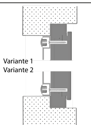
Montage A - einfache Tür
